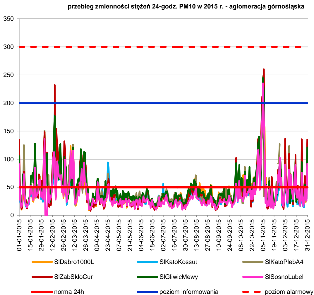
Rysunek 8. Przebieg zmienności stężeń dobowych pyłu zawieszony PM10 w 2015 roku w strefie aglomeracja górnośląska 63
